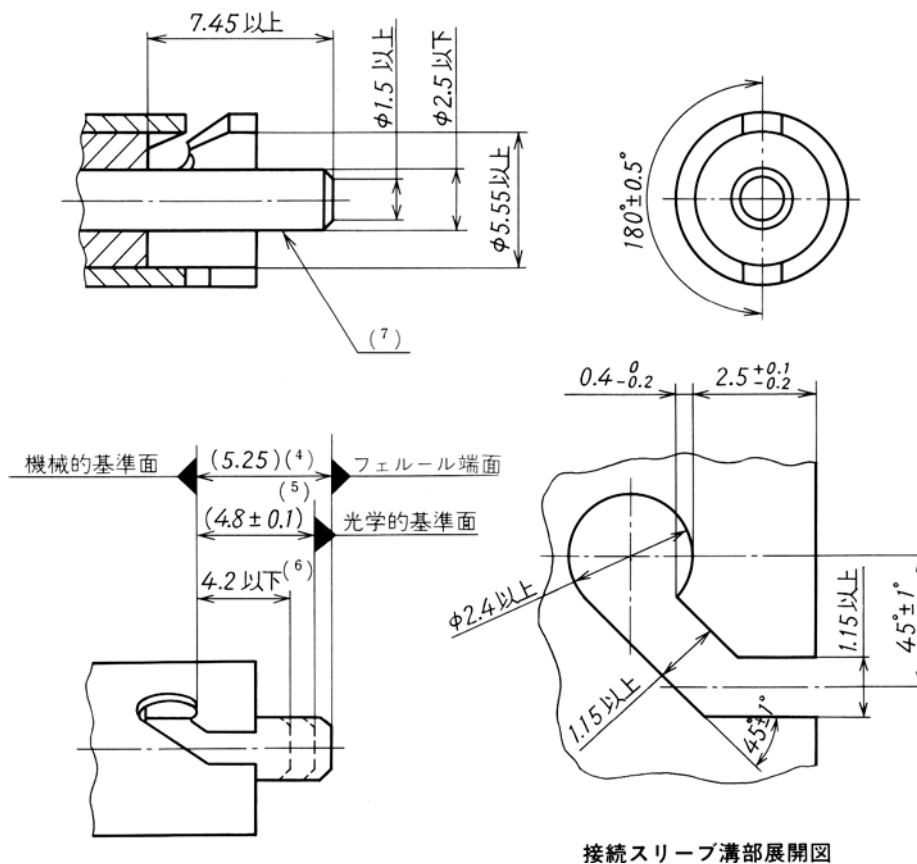
図 1 光コネクタ結合部 (プラグ)
