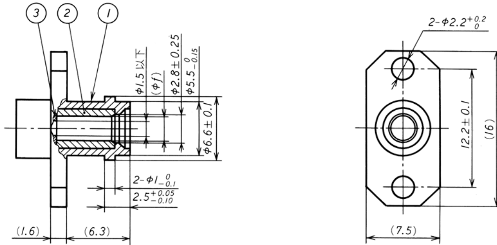
付図 6 光コネクタの形状及び寸法 (CNF09DRF-1)
