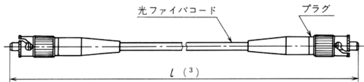
参考 2 図 1 コード付き光コネクタの形状及び寸法
