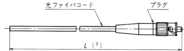
参考 2 図 3 コード付き光コネクタの形状及び寸法
