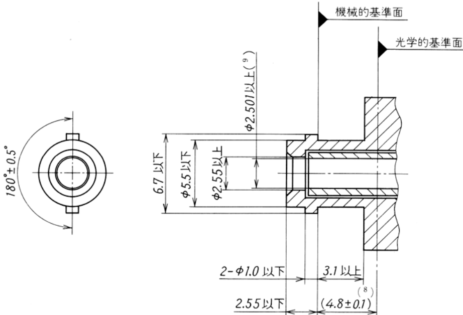
図2 光コネクタ結合部 (アダプタ)
