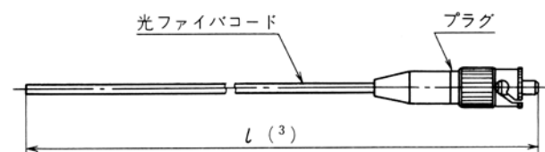
参考 2 図 4 コード付き光コネクタの形状及び寸法
