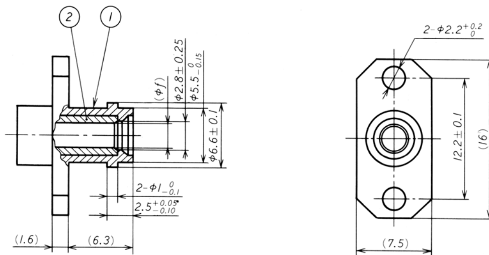
付図7 光コネクタの形状及び寸法 (CNF09DRF-2)
