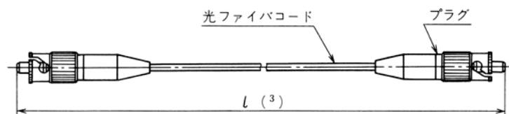
参考 2 図 3 コード付き光コネクタの形状及び寸法
