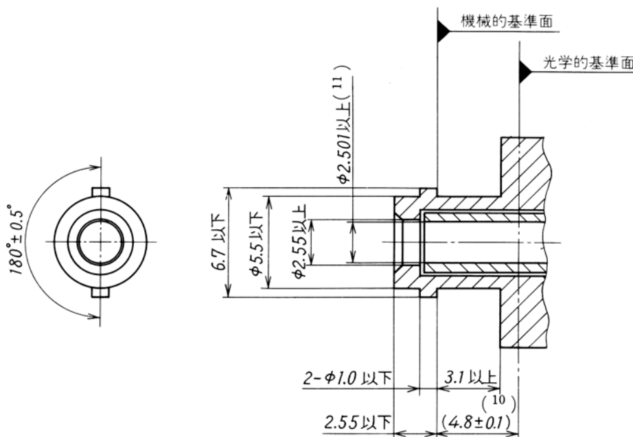
図3 光コネクタ結合部 (レセプタクル)
